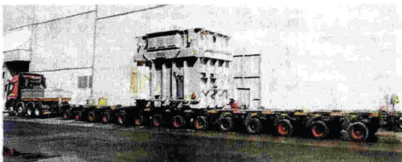
Ecco uno dei trasformatori posizionato sul mezzo della FT International
